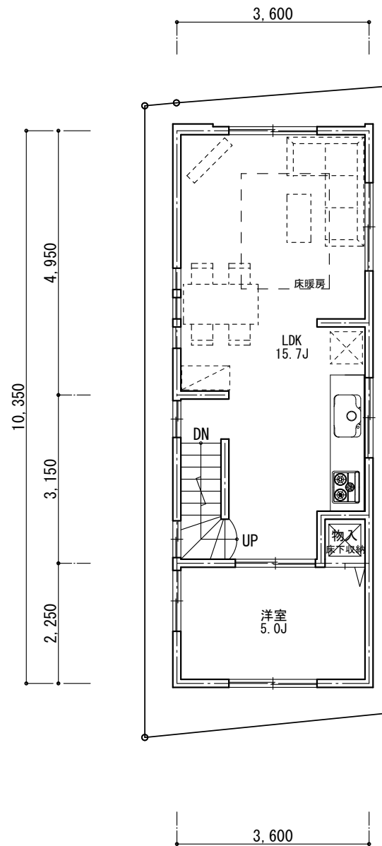
2階平面図 S=1/100
