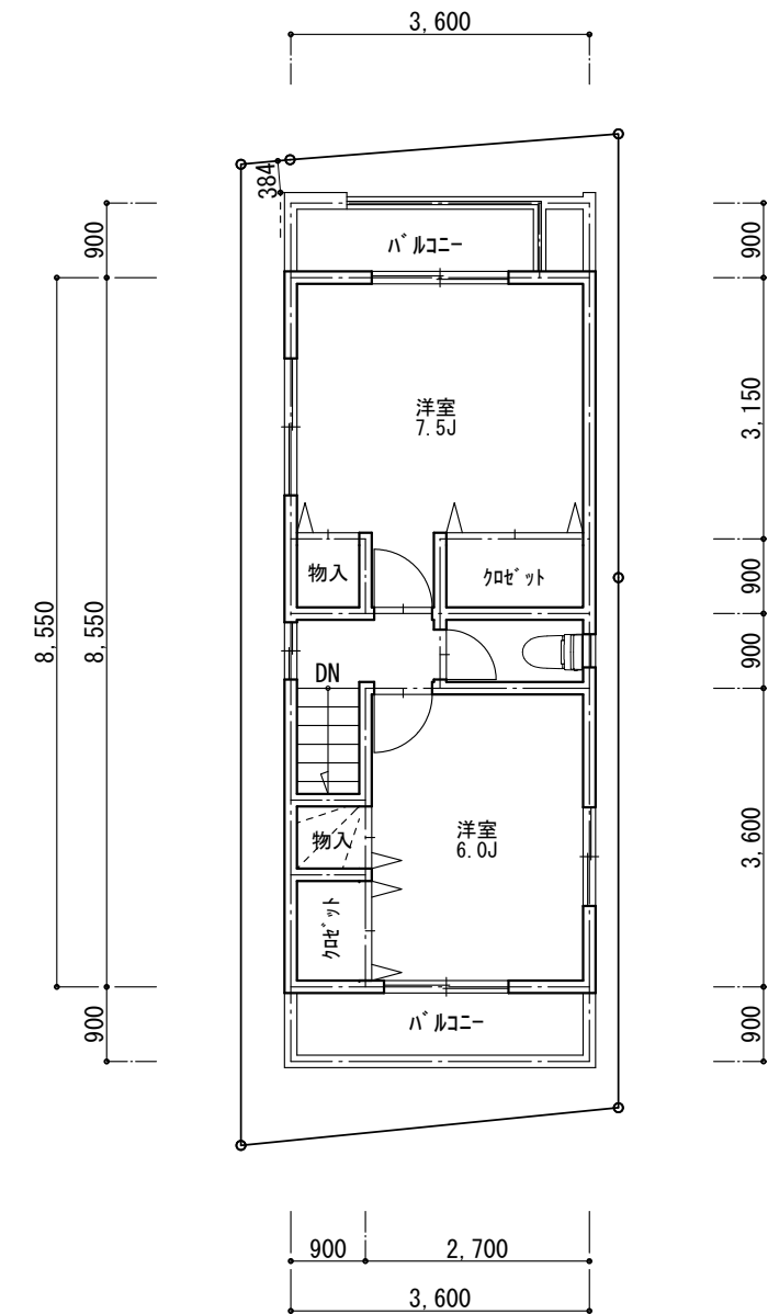
3階平面図 S=1/100
