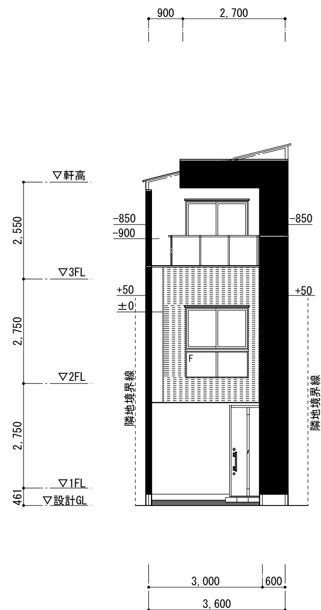
北立面図 S=1/100
