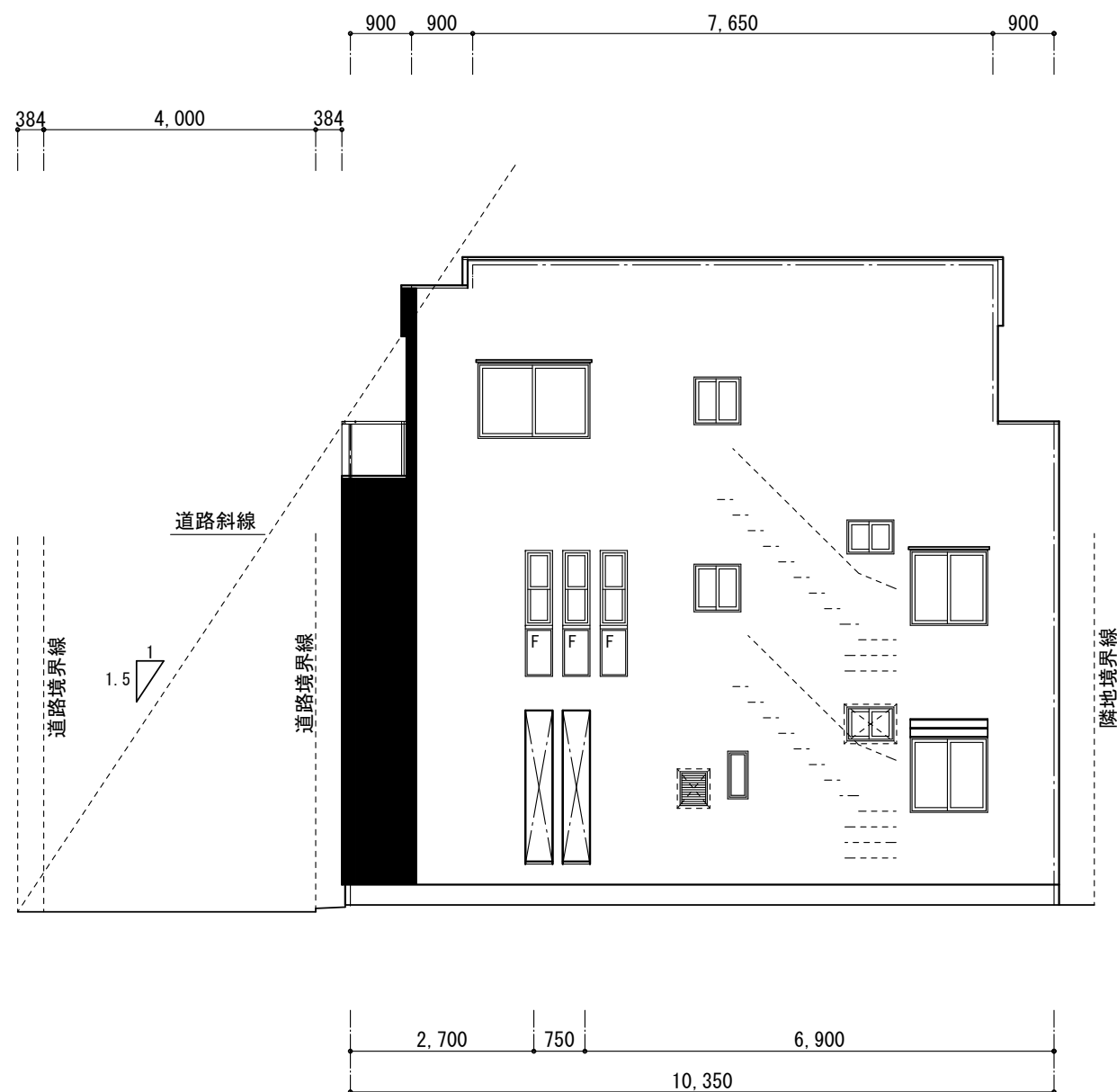
西立面図 S=1/100
