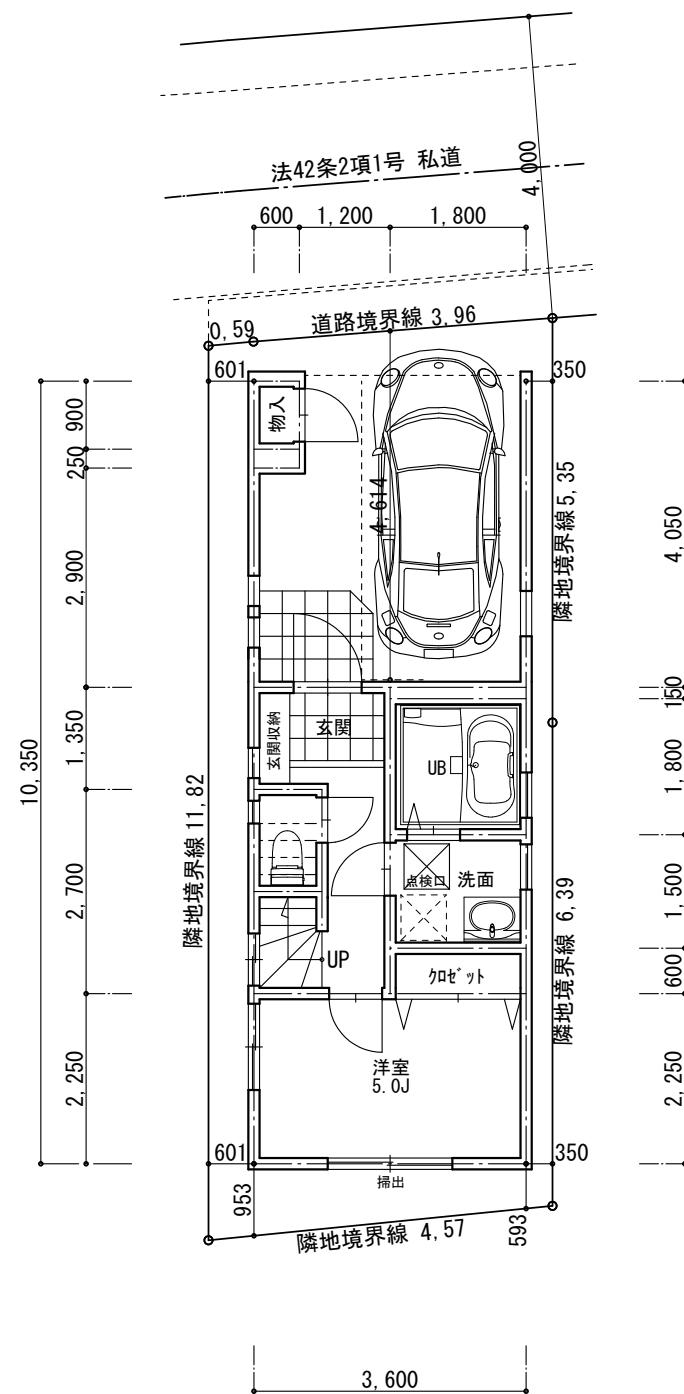
1階平面図 S=1/100
