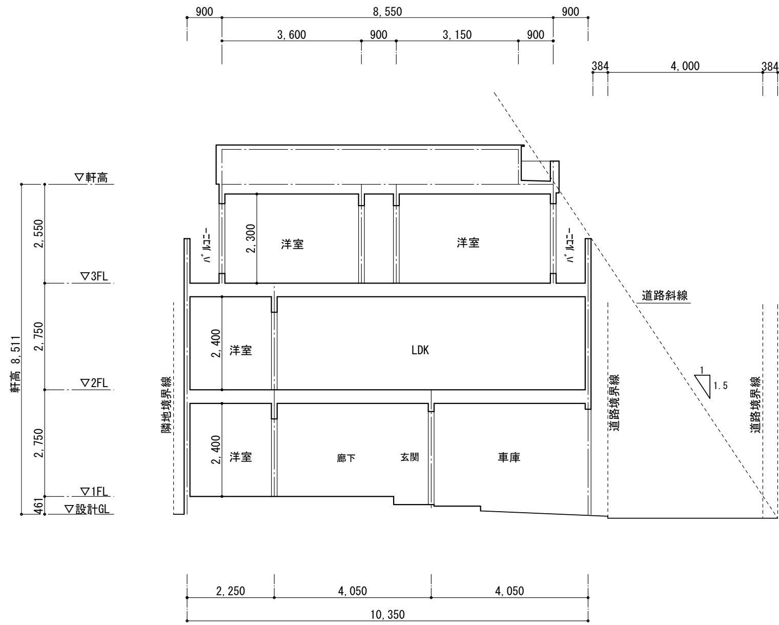
断面図 S=1/100
