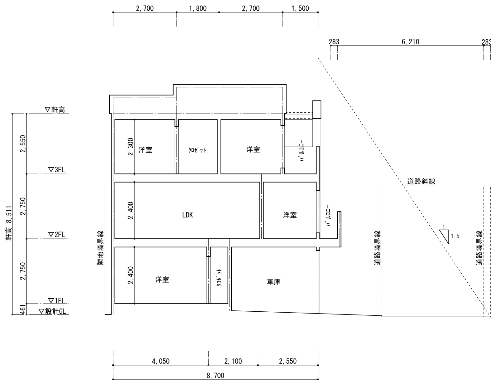
断面図 S=1/100
