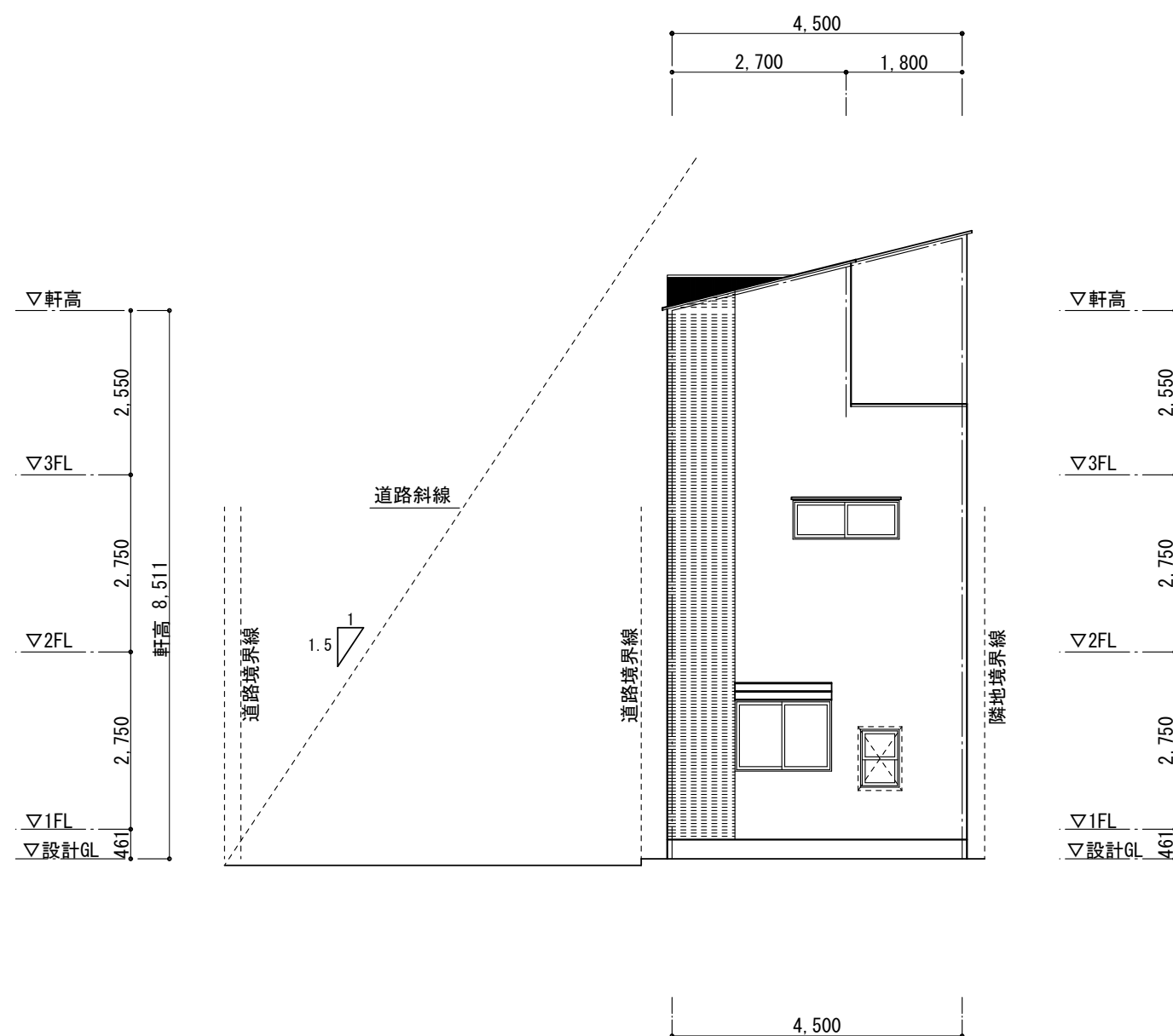
西立面図 S=1/100
