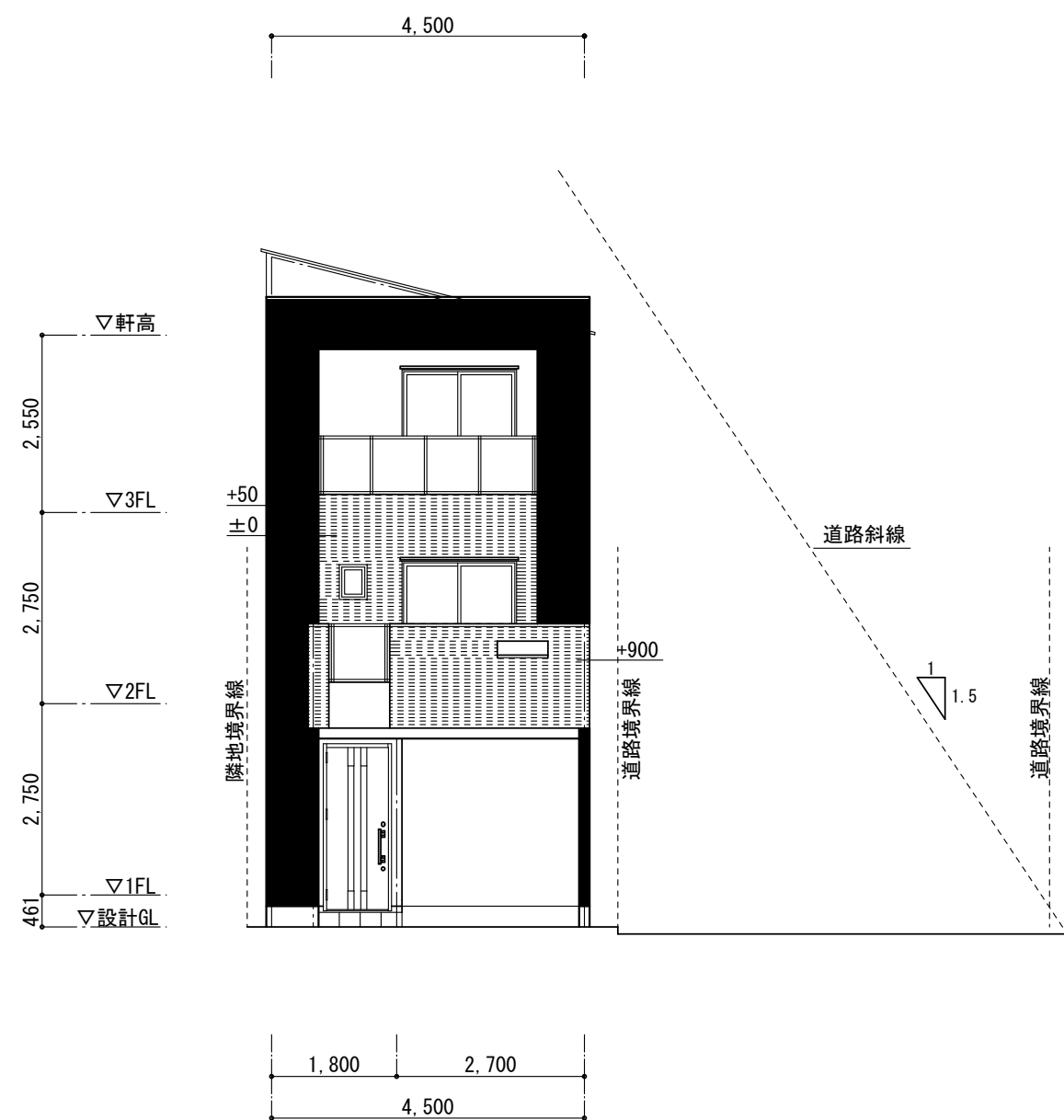
東立面図 S=1/100
