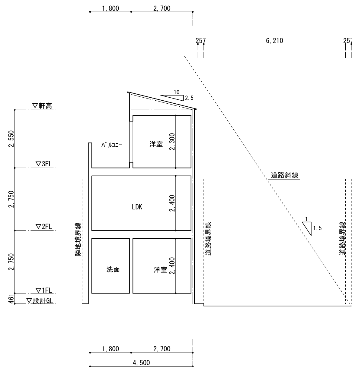
断面図 S=1/100
