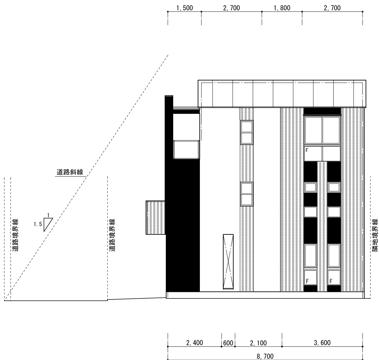
北立面図 S=1/100
