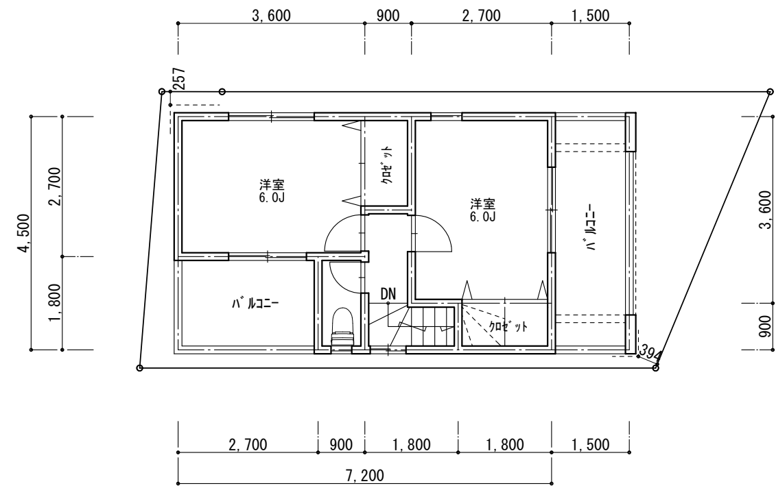
3階平面図 S=1/100
